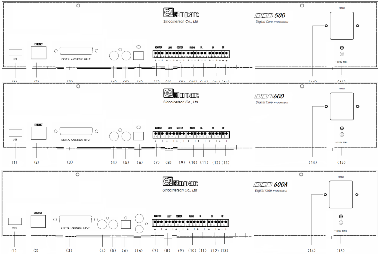
图4-1 DCP500/600/600A型数字电影音频处理器背板与设备连接图
