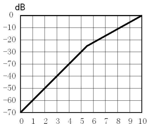
图 3-2 主音量控制增益输出特性
