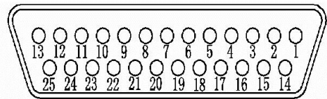
图 4-2 6 声道数字输入信号接口
