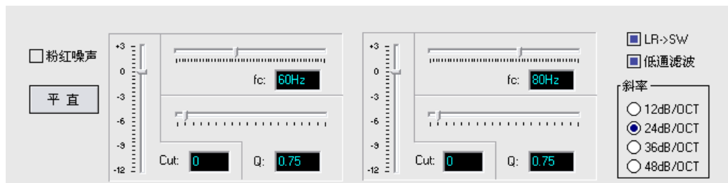
图 5-16 次低频参量均衡界面
