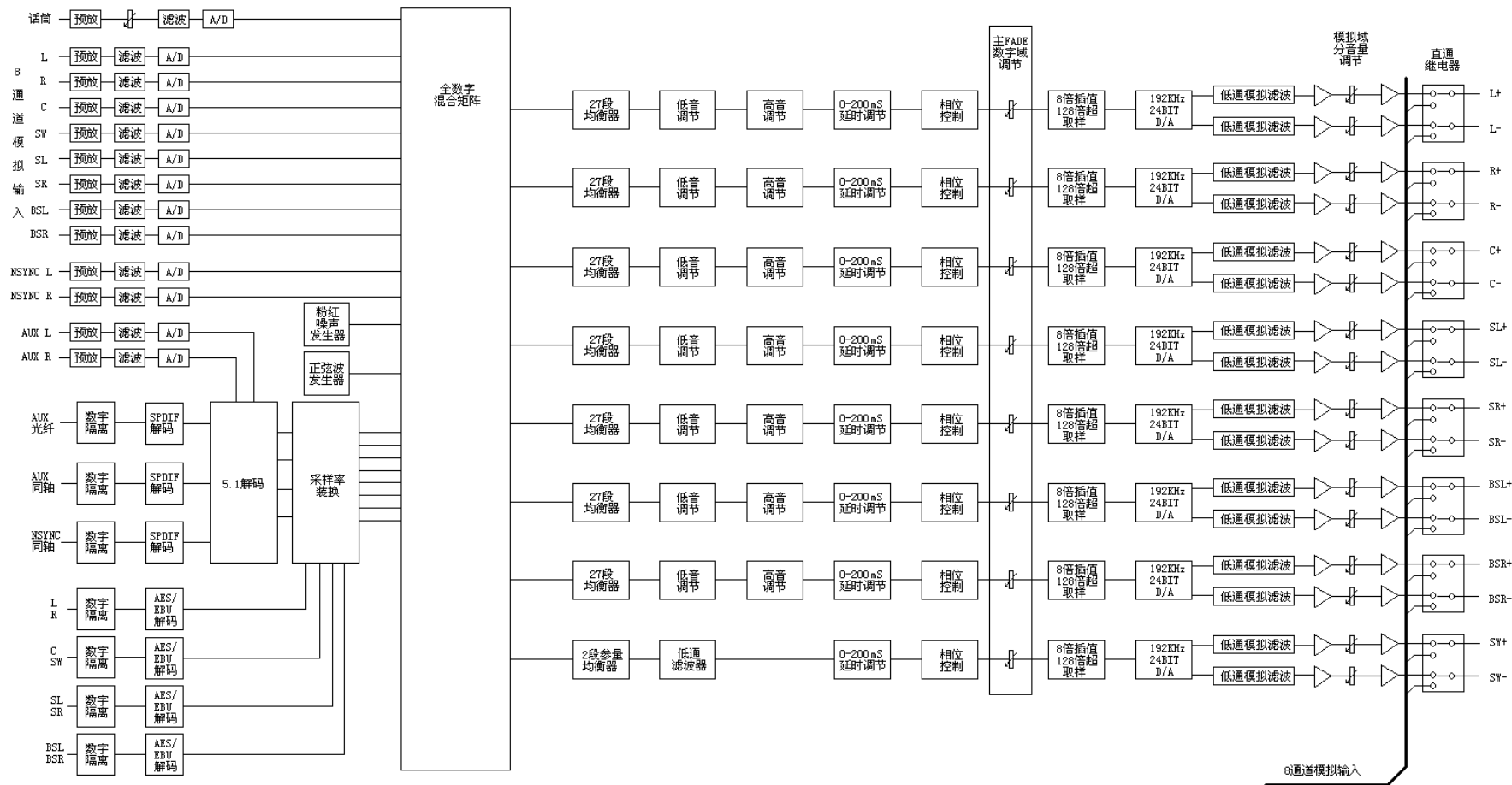
图 2-1 DCP500/600/600A 数字电影声频处理器系统框
