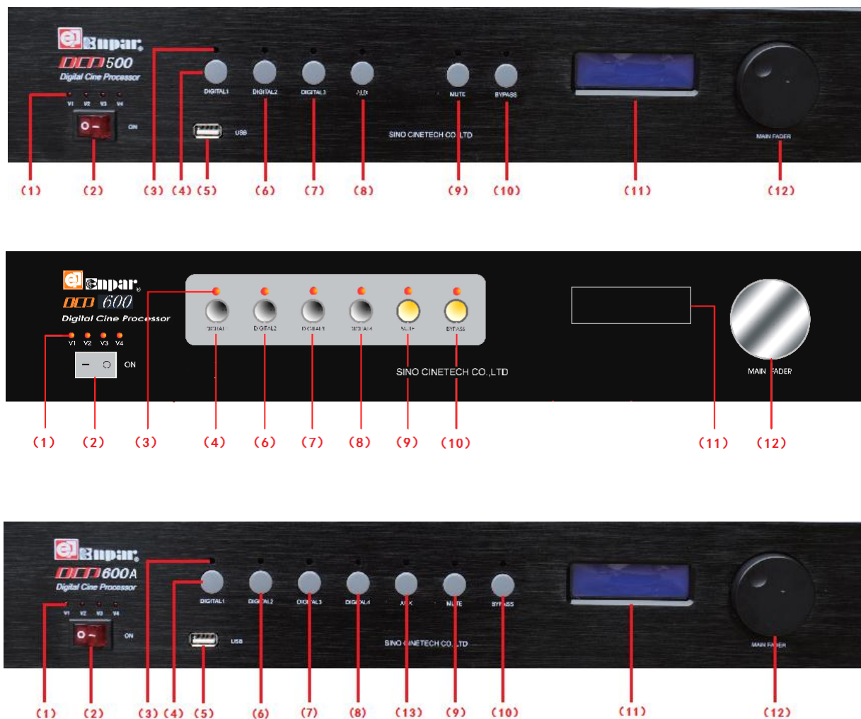
图3-1 DCP500/600/600A型数字电影声频处理器前面板
